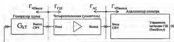
Рисунок 1б. Измерение суммарного коэффициента шума четырехполюсника в анализатор спектра КШ чпвас
